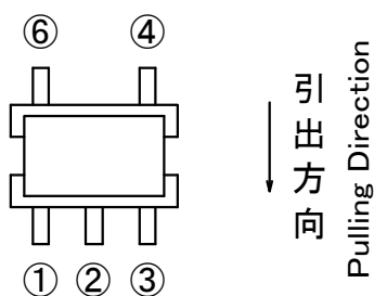
上面図 Top view
